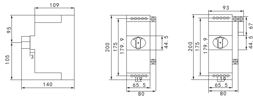
控制保护开关-45标准尺寸 (图3)
